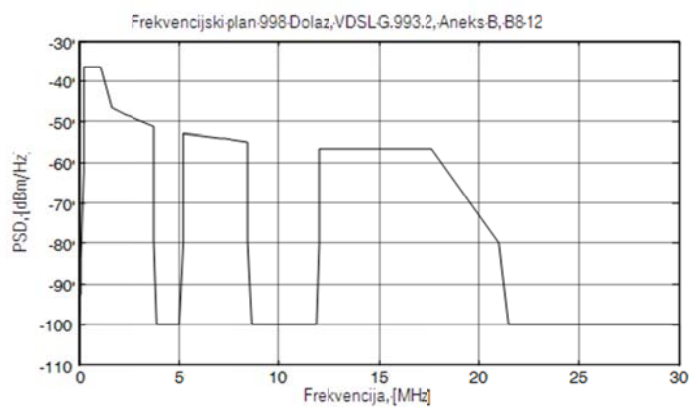
Slika 5.5.1 Frekvencijski predložak za VDSL2 frekvencijski plan 998, B8-12 dolaz (crno).
